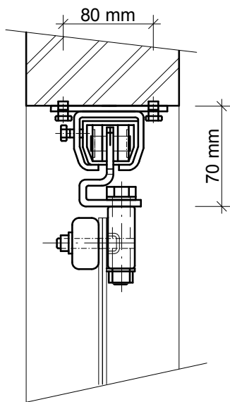
POSUVNÁ TYP A (do světlosti otvoru)
