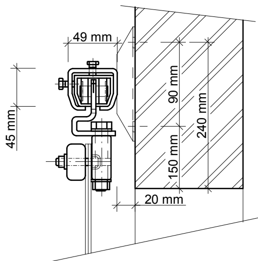
POSUVNÁ TYP B (nad světlost otvoru)
