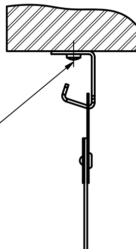
Hřebenová lišta - Typ A (do světlosti otvoru)
