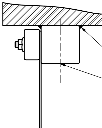
Svěrná lišta - Typ A (do světlosti otvoru)
