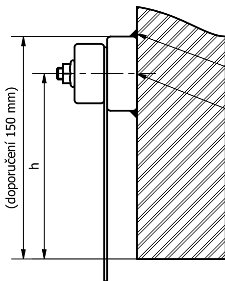
Svěrná lišta - Typ B (nad světlost otvoru)
