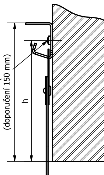
Hřebenová lišta - Typ B (nad světlost otvoru)
