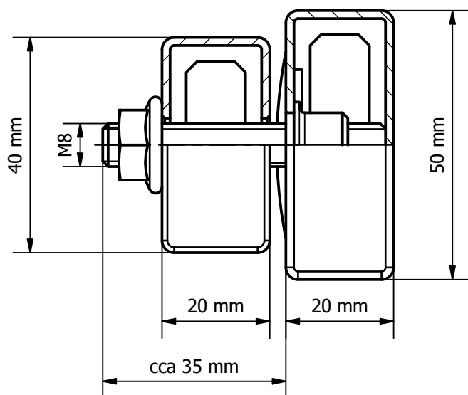
Detail svěrné lišty s přítlačným profilem (1:1)
