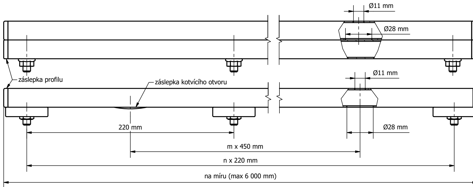
Detail svěrné lišty s přítlačným profilem (1:1)
