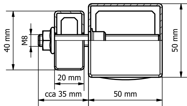
Detail svěrné lišty s přítlačným profilem (1:1,5)
