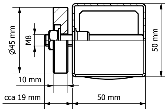
Detail svěrné lišty s plastovými podložkami (1:1,5)
