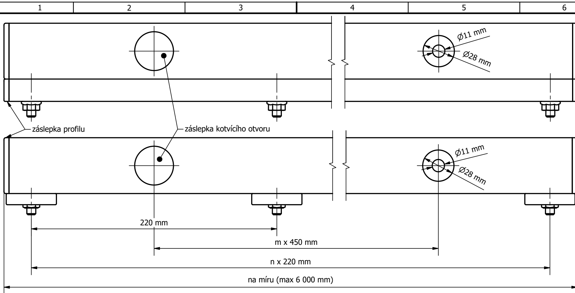
Detail svěrné lišty s přítlačným profilem (1:1,5)
