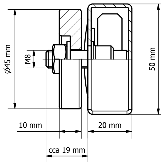
Detail svěrné lišty s plastovými podložkami (1:1)
