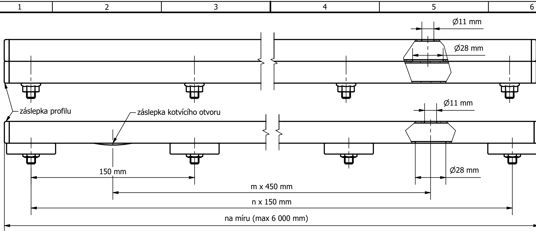
Detail svěrné lišty s přitlačným profilem (1:1)
